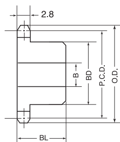
B型 (材質機械構造用炭素鋼) 35Tまで鍛造品ヤキナシ
