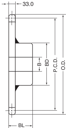
BW型 (SS400) SS400 溶接品
