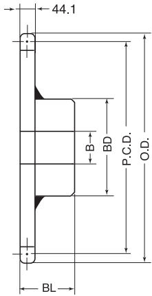
BW型 (SS400) 溶接品
