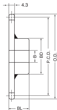
新BW型 (材質SS400) 41T～溶接品
