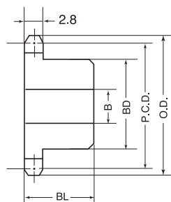
B 型 (機械構造用炭素鋼)
