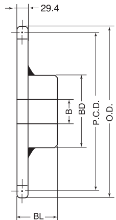
新BW型 (SS400) 21Tまで 歯部機械構造用炭素鋼 ボスSS400 溶接品 22T～溶接品
