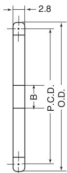
A型 (材質SS400) 酸洗材プレス抜
