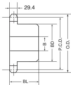
新B型 12Tまで機械構造用炭素鋼 鍛造品
