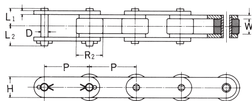
Rローラ型
