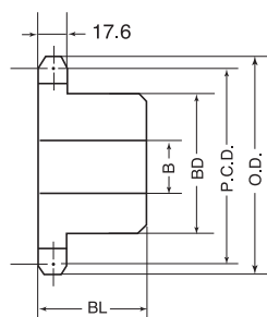
新B型 (材質機械構造用炭素鋼) 21Tまでヤキ入鍛造品
