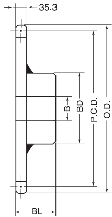
BW型 (SS400) SS400 溶接品
