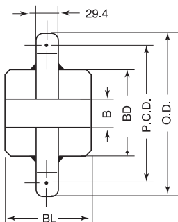
C型 SS400 溶接品
