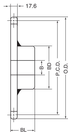
新BW型 (材質SS400) 22T～溶接品
